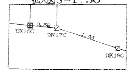
拡大図S=1:50
